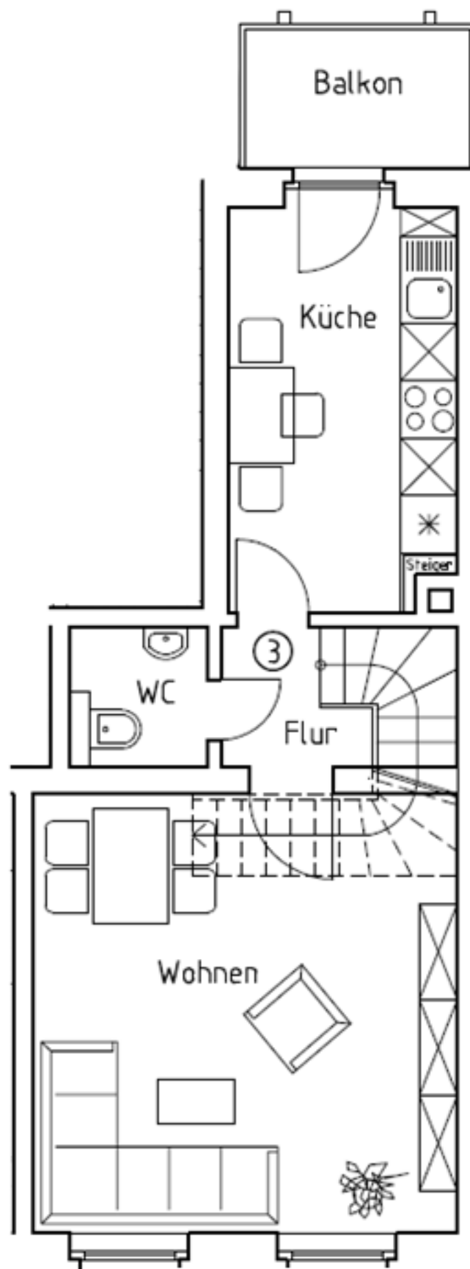
1. Obergeschoss
